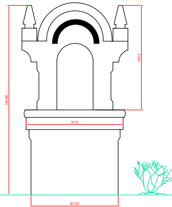
Estado reformado
